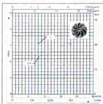
CURVA DE DESEMPENHO
